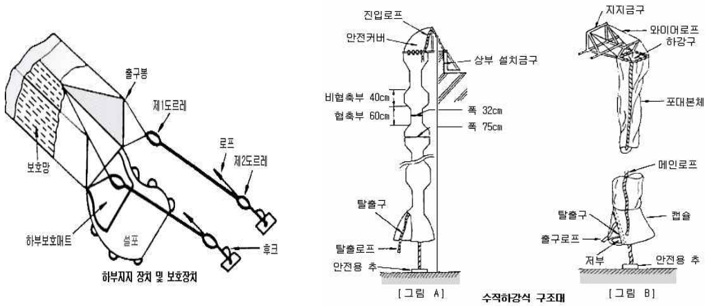
▲ 경사하강식 구조대
