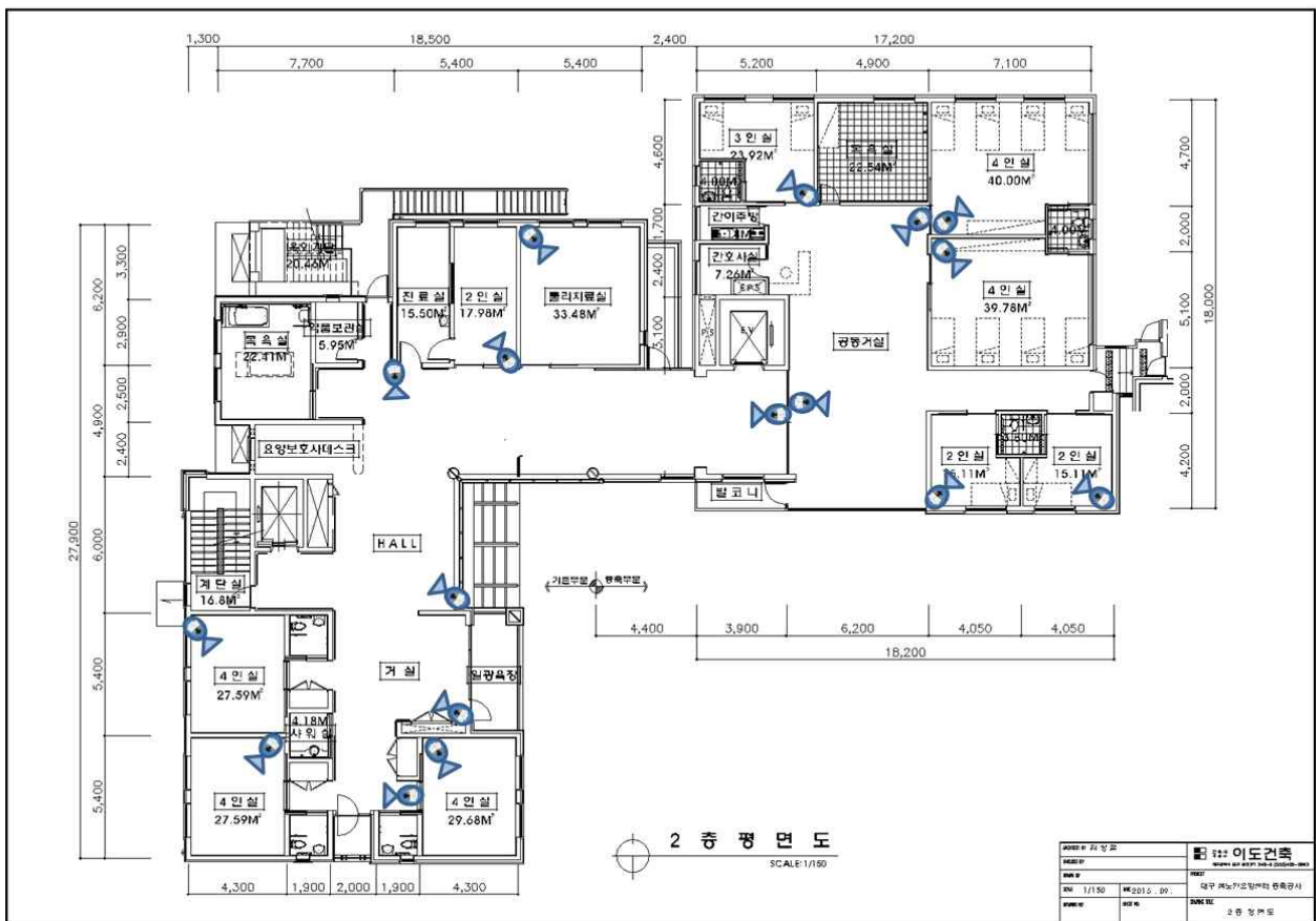
2층 CCTV 설치 준공도면 – 17채널(1개채널 1층 NVR연결)
