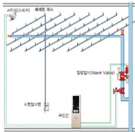
▲ 계통도
