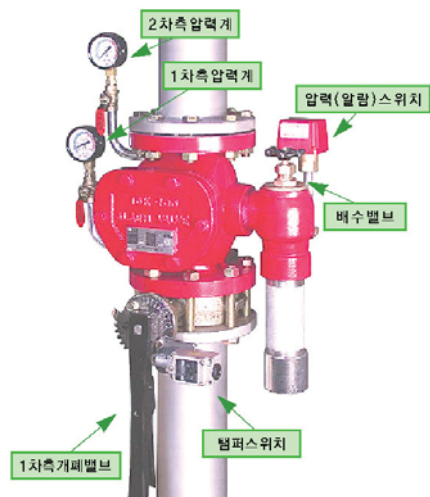
▲ 유수검지장치
